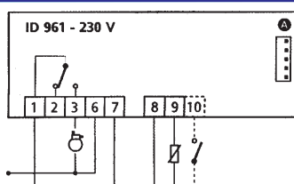
ID 961/A NTC
